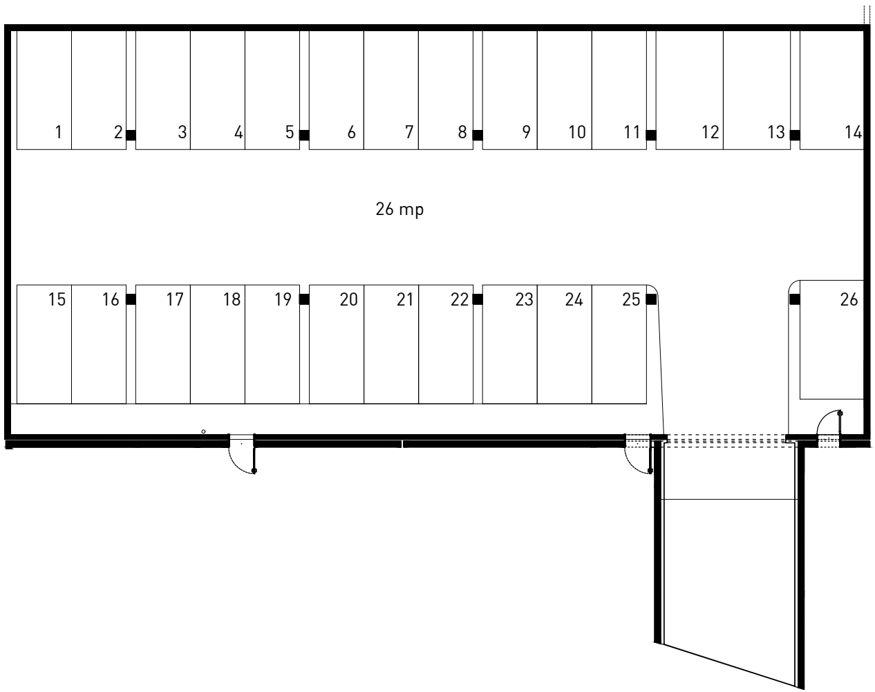
PARKING _ KONDYNACJA -1 _ KUŹNIKI _ BUDYNEK B
